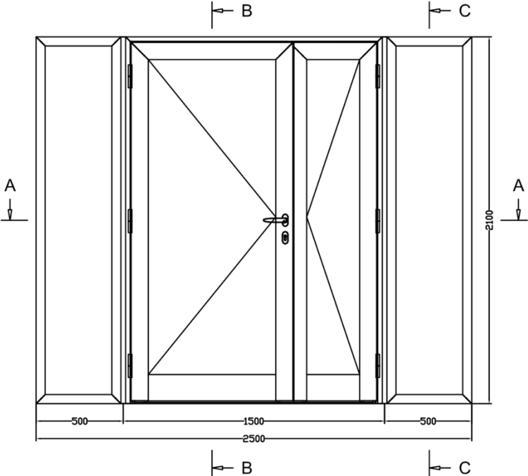
Élévation 1 - Vue extérieure
