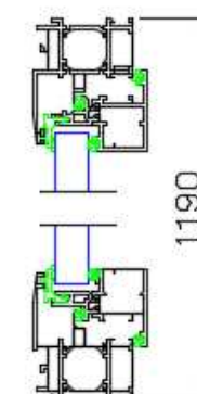
Coupe B-B
