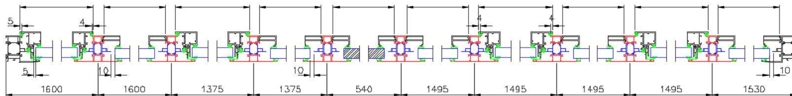
Coupe A-A
