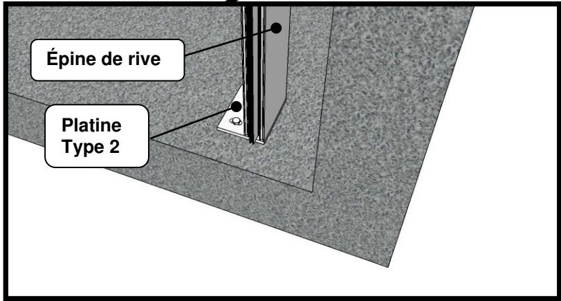
Détail de la fixation de l'épine de rive au plancher et au plafond
