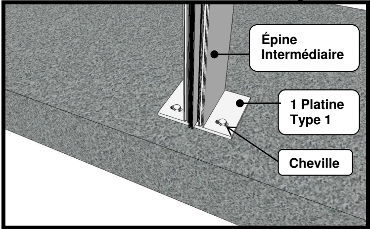
Détail de la fixation de l'épine intermédiaire au plancher et au plafond
