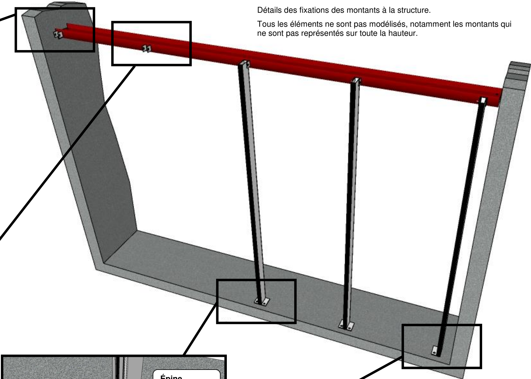
Vue partielle 3D du mur-rideau MR01 en cours de réalisation
