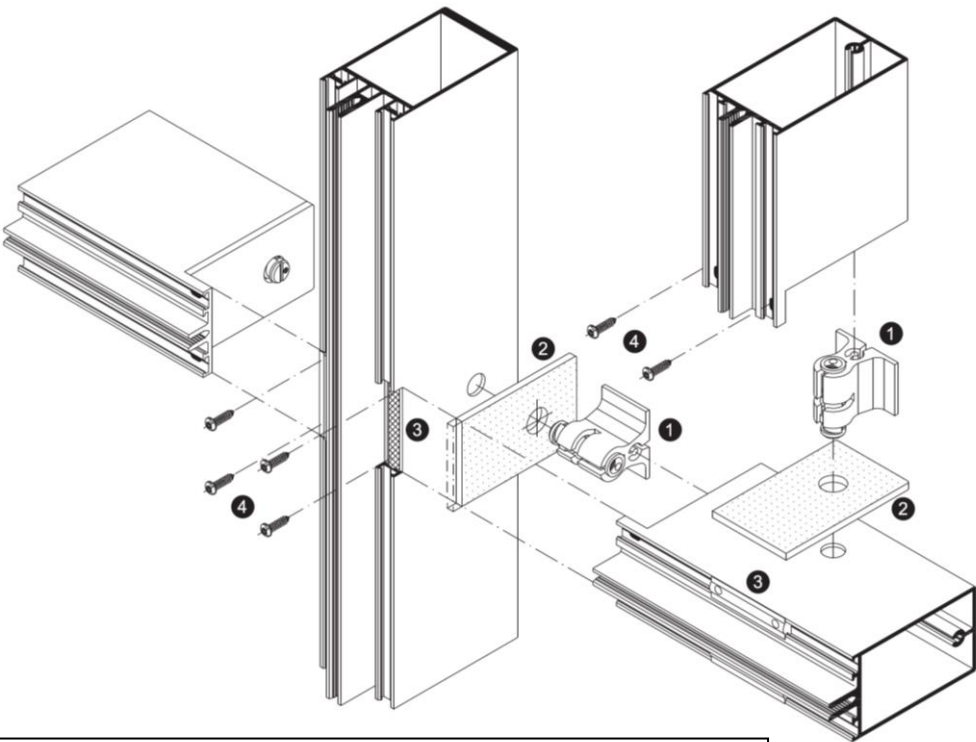
PERÇAGE POUR ASSEMBLAGE
